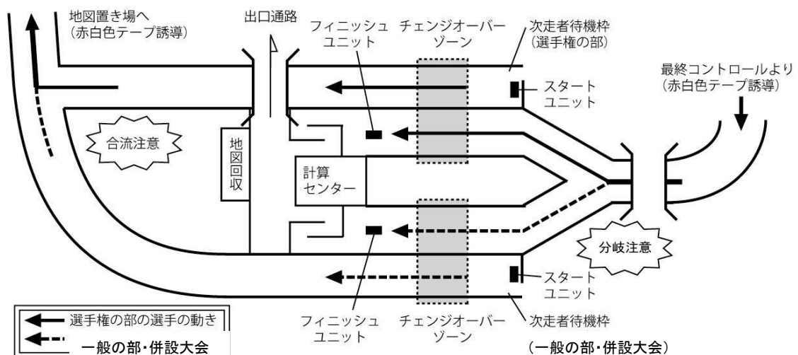
<スタート/フィニッシュ地区レイアウト図>
